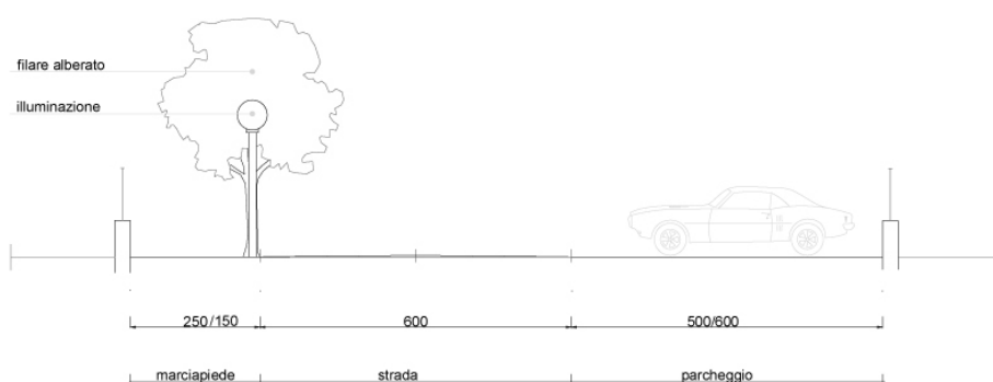
Fig 1: Sezione stradale e di arredo urbano tipo
